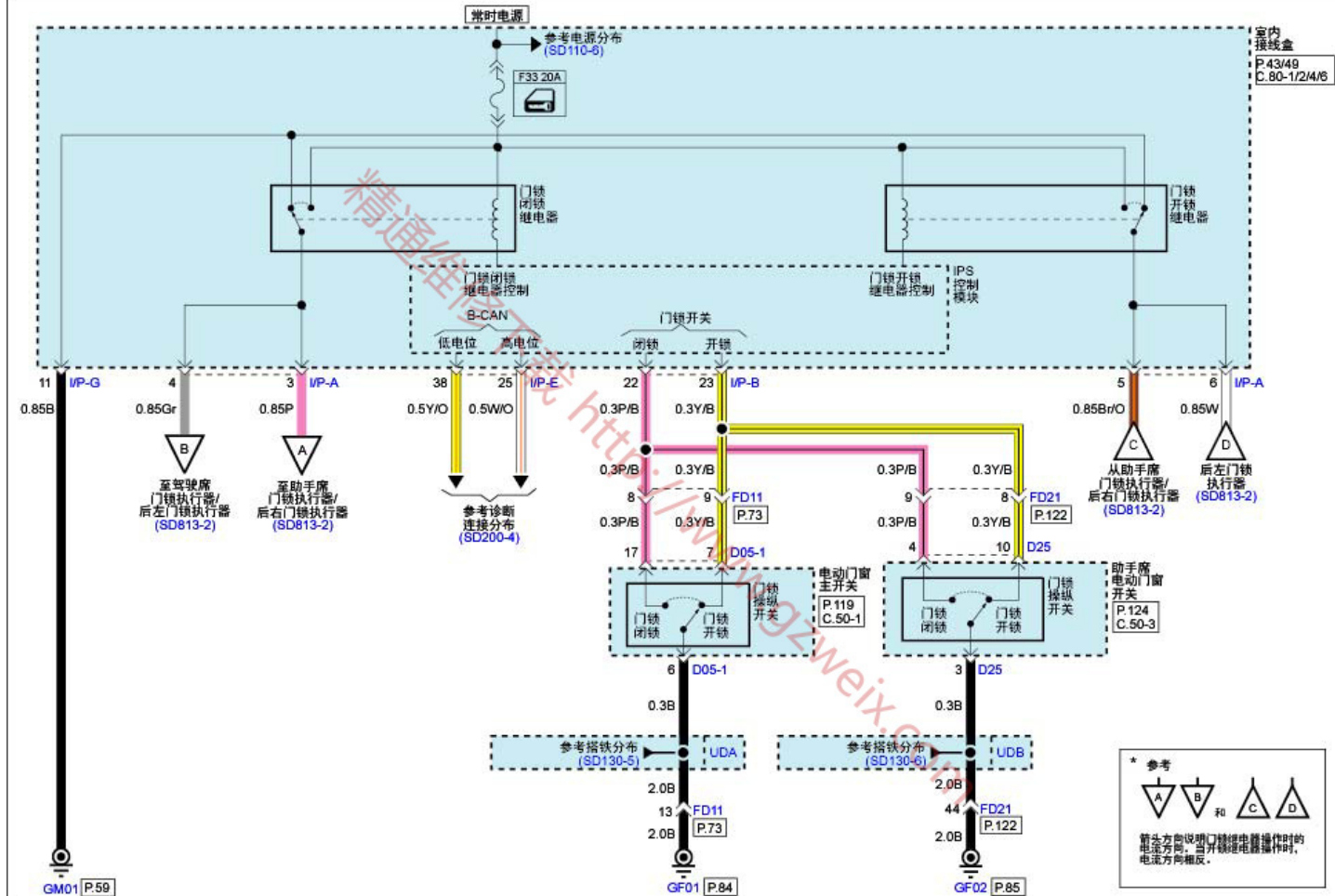
电动门锁(1)
